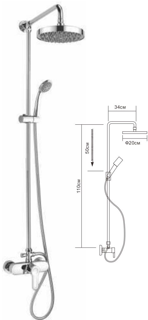
D10A07 Латунь Душевая система со смесителем
